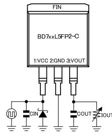
TO263-3F
